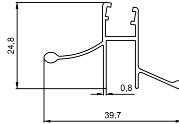
J 1105 0,238 Kg/m
