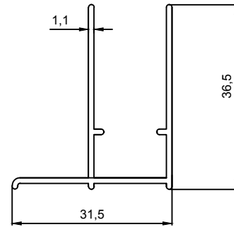
J 1250 0,319 Kg/m
