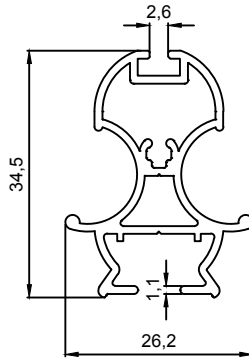
J 1257 0,443 Kg/m
