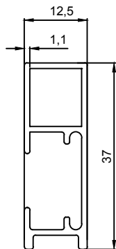
J 1249 0,446 Kg/m
