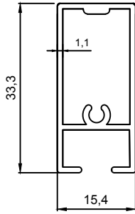
J 1256 0,338 Kg/m
