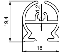
J 1258 0,267 Kg/m
