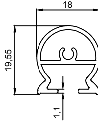
J 1252 0,254 Kg/m
