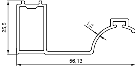
J 1247 0,448 Kg/m
