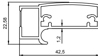
J 1873 0,492 Kg/m
