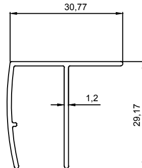
J 1250 0,319 Kg/m
