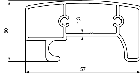
J 2087 0,797 Kg/m
