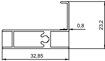
J 1104 0,255 Kg/m
