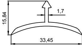
J 1091 0,217 Kg/m
