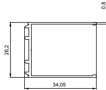
J 1105 0,238 Kg/m
