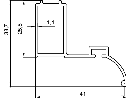
J 1248 0,365 Kg/m
