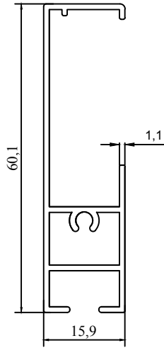
J 1249 0,446 Kg/m
