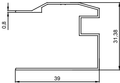
J 1106 0,282 Kg/m
