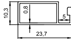
J 1031 0,153 Kg/m
