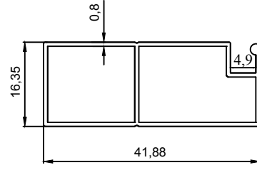
J 1027 0,294 Kg/m
