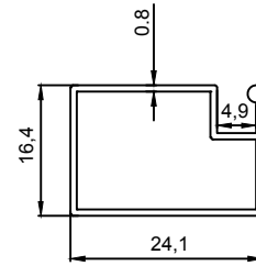
J 1034 0,186 Kg/m
