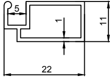
J 1000 0,178 Kg/m
