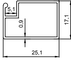
J 1001 0,238 Kg/m
