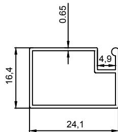
J 1034-B 0,165 Kg/m
