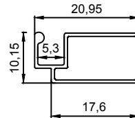
J 1594 0.120 Kg/m
