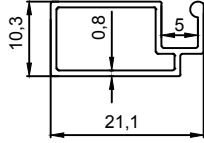
J 1030 0,141 Kg/m
